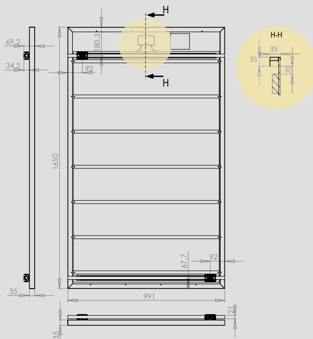
Plan du panneau Spring version non-isolée avec raccord DualQuickfit® DN15
